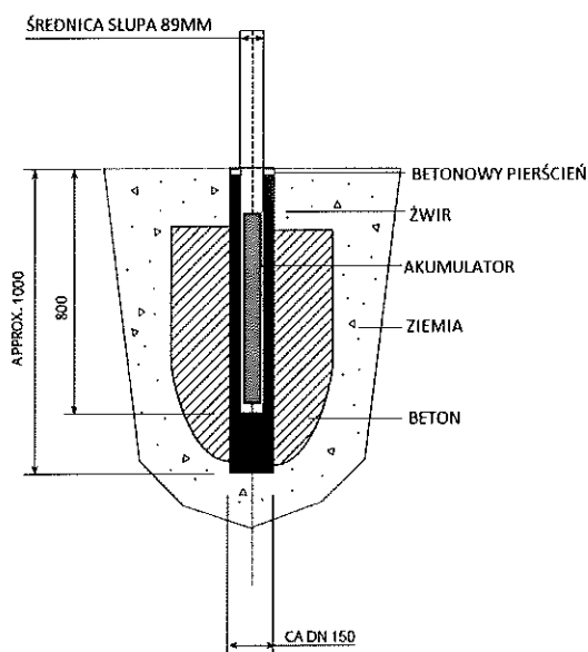
Fundament
